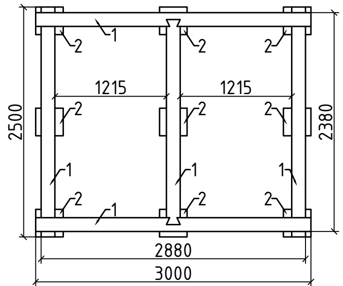
План фундамента
